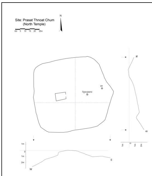
ប្លង់ប្រាសាទត្នោតជុំខាងជើង (គុកជើង)
