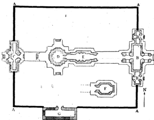
Fig. 119. — Prasat Kuk Nokor, n° 147. Plan. (Échelle 1/500.)
