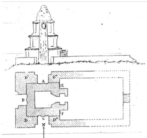
ប្លង់ប្រាសាទត្នោតជុំខាងជើង (គុកខាងជើង)
